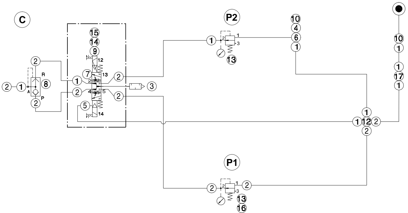
Schema 0562.1986.3
